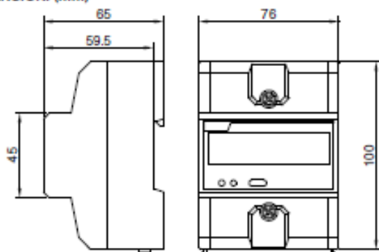
DIMENSIONI (mm)
