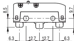
Terminali vite V con piastrina
