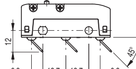
Terminali a faston F , piega DX
