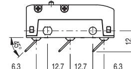
Terminali a faston G , piega SX (a richiesta)
