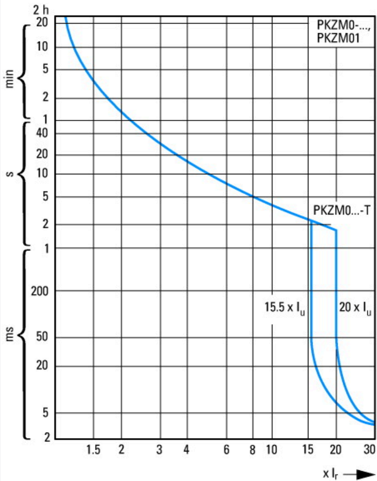
Curve caratteristiche d'intervento interruttore protettore partenza motore compatta (ad alte prestazioni), PKZM0-...T (non per PKM0-...), PKZM01
